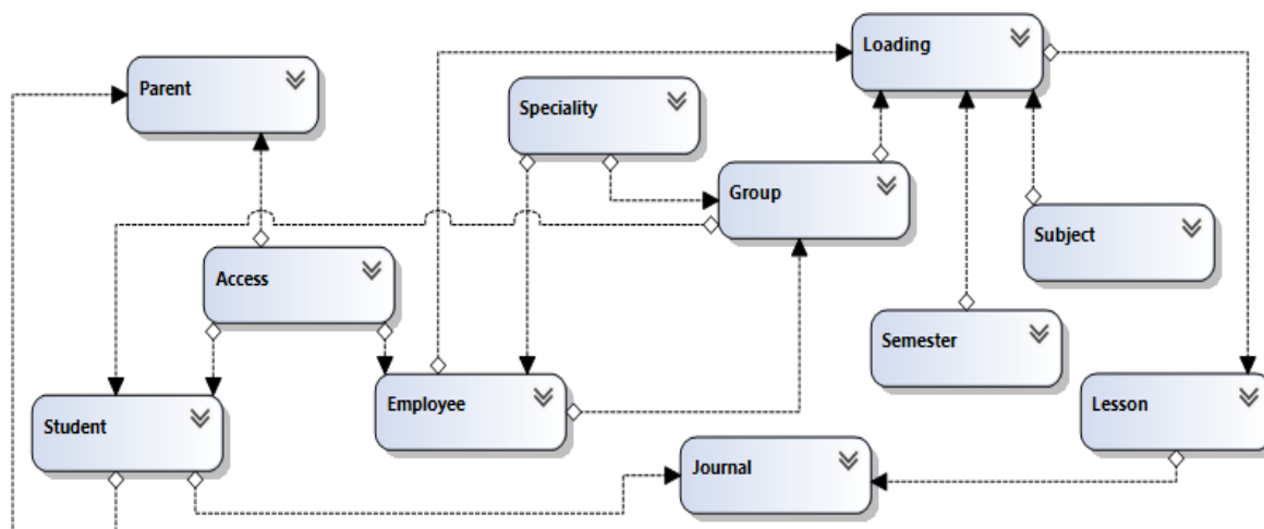
Рисунок 3 – Діаграма .NET класів веб-сервісу організації навчального процесу
