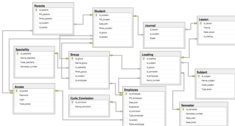
Рисунок 2 – База даних веб-сервісу організації навчального процесу
